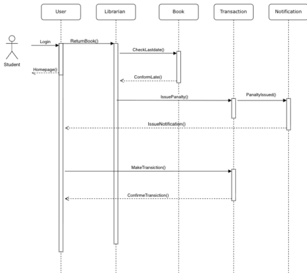
SequenceDiagram2:
